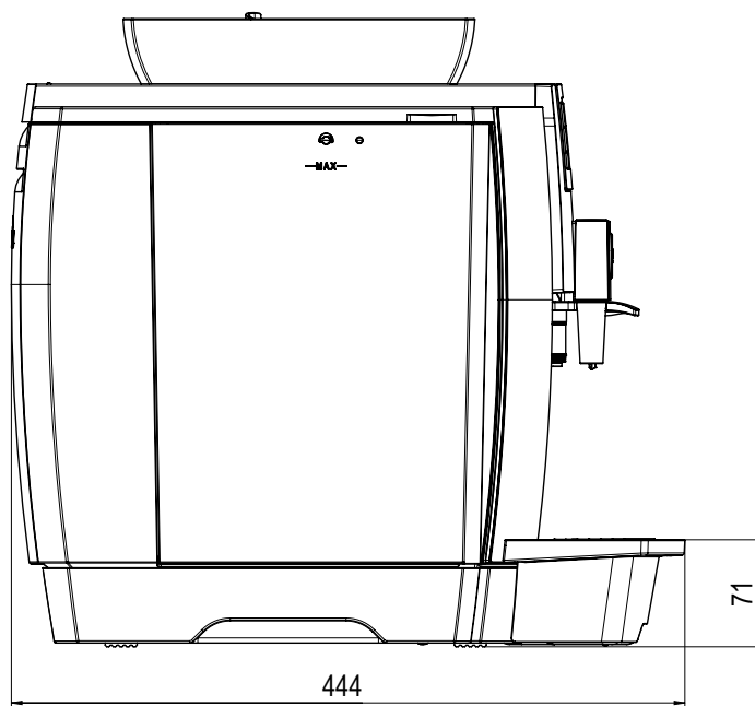
Zijaanzicht
